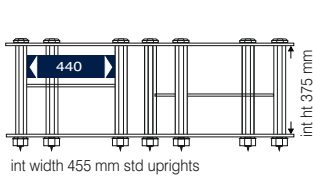
Ultimate AV Support (hwd 440 x 1322 x 600)
